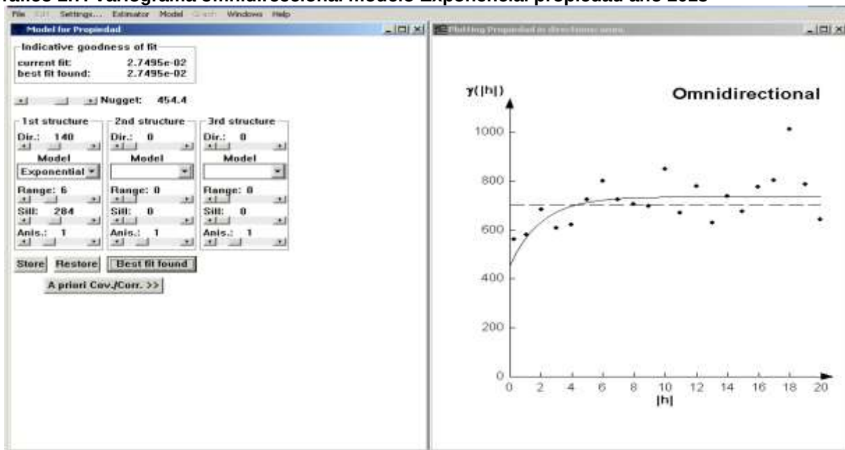
Gráfico 2.7. Variograma omnidireccional modelo Exponencial propiedad año 2013
