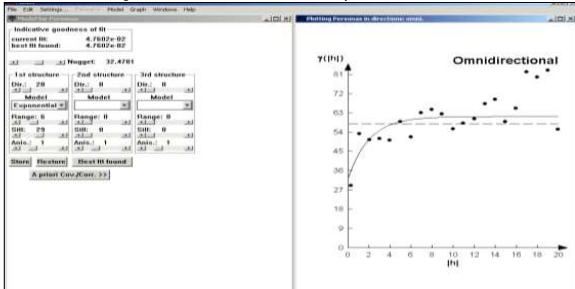
Gráfico 2.16. Variograma omnidireccional modelo Exponencial
