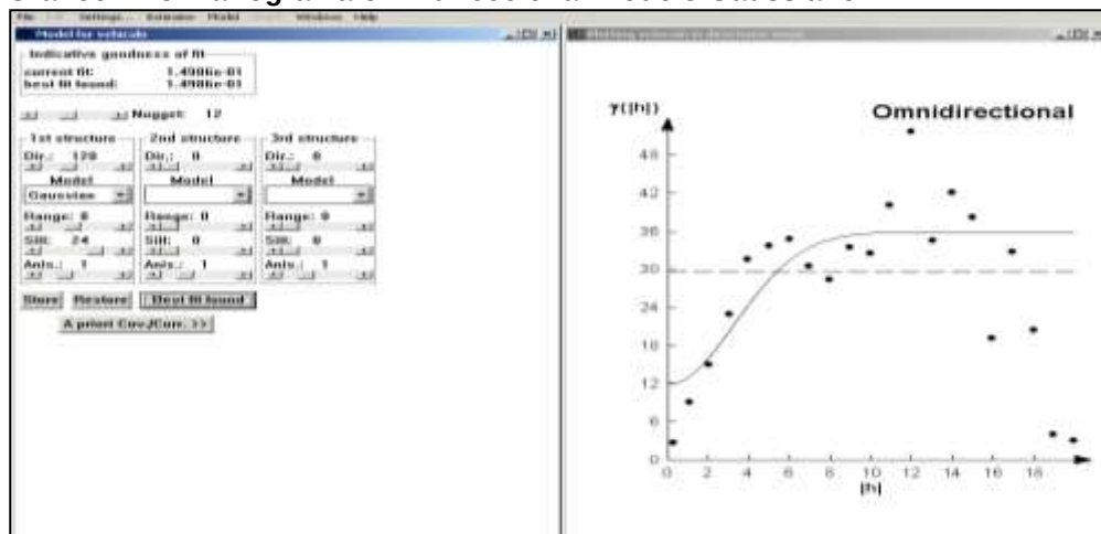
Gráfico 2.13. Variograma omnidireccional modelo Gaussiano
